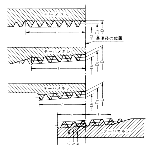
付表 テーパオネジとテーパメネジまたは平行メネジとののはめあい
