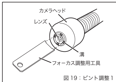
図 19：ピント調整 1
