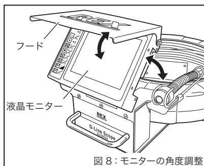
図8: モニターの角度調整
