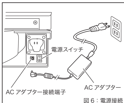
図 6：電源接続
