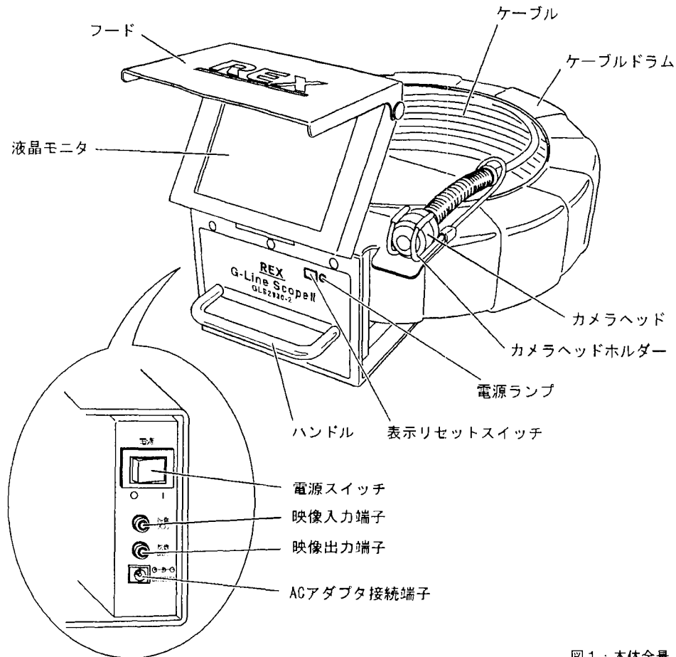
図1：本体全景
