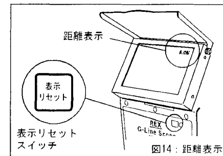
図14: 距離表示
