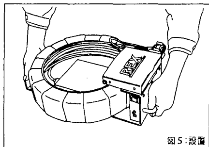
図5: 設置
