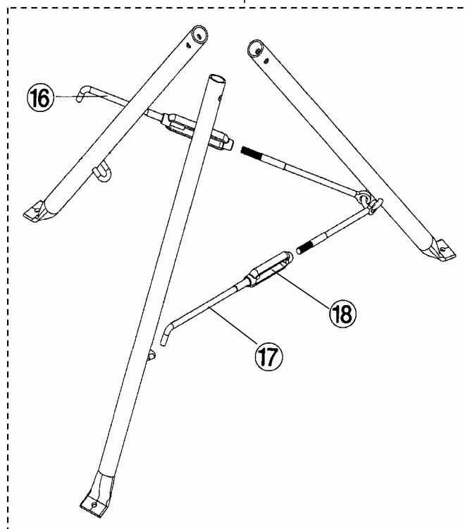
VL1 Leg
